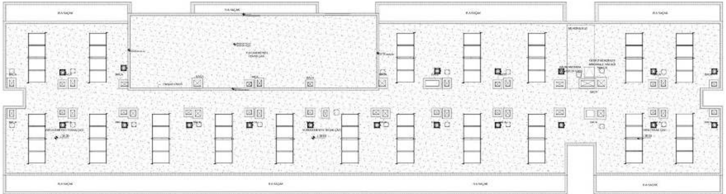
Çatı Planı
