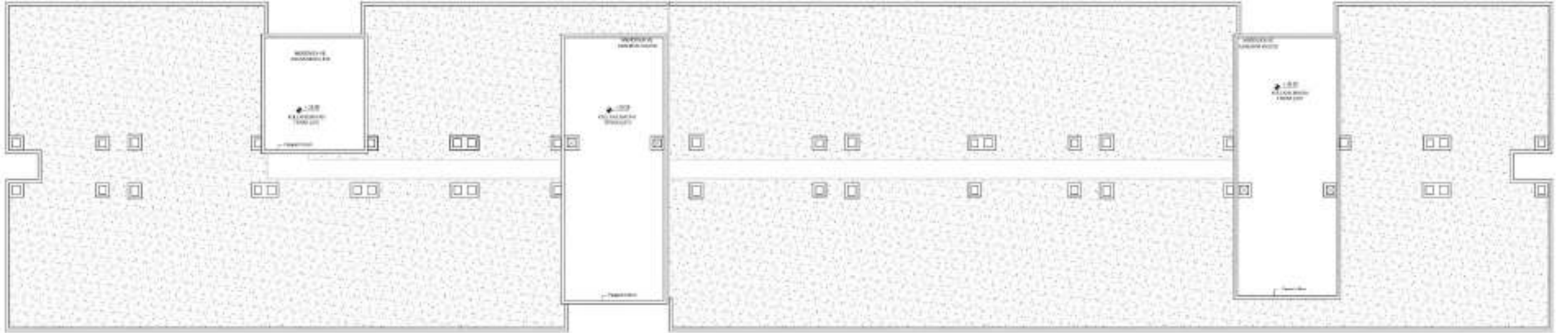
Çatı Planı
