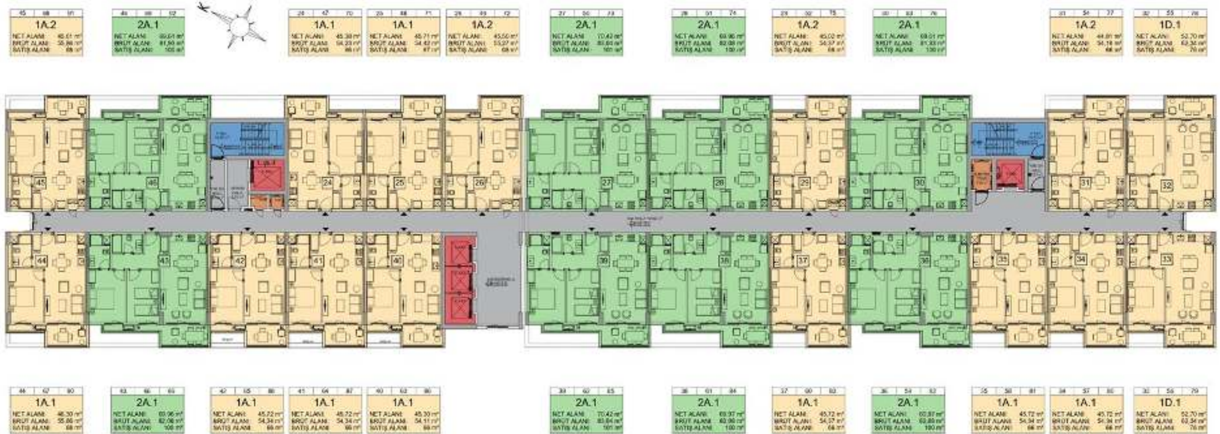
3-4-5. Kat Planı
